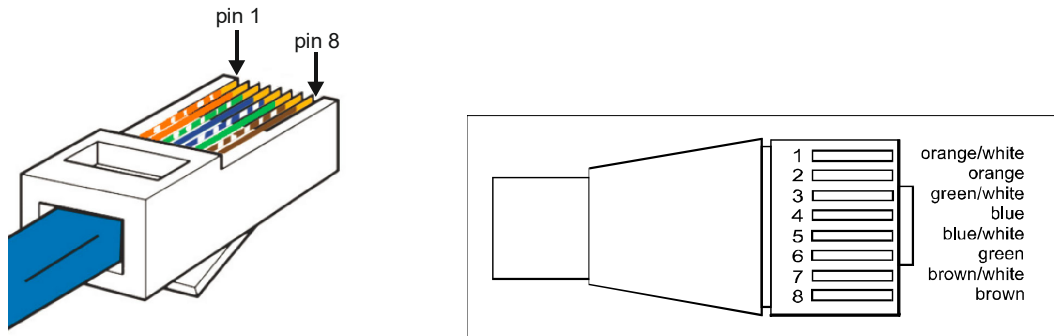
Dettaglio intestazione cavo su plug RJ45
